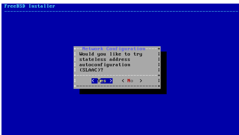
図2.38 IPv6 SLAAC 設定の選択
