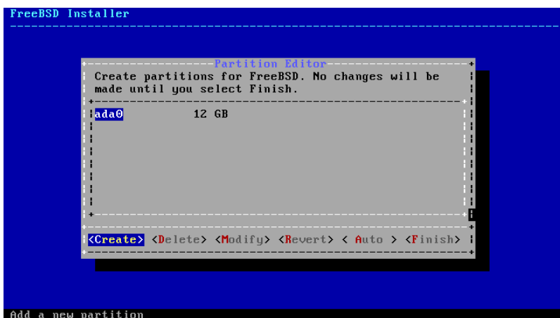
図2.15 Manual によるパーティションの分割
