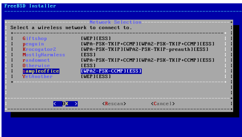
図2.32 ワイヤレスネットワークの選択
