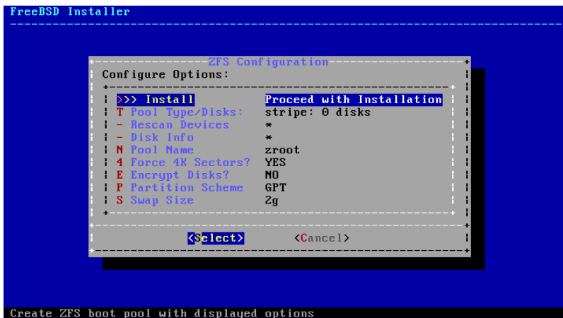
図2.18 ZFS パーティションメニュー
