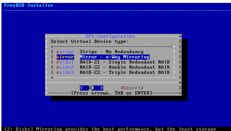
図2.19 ZFS プールタイプ
