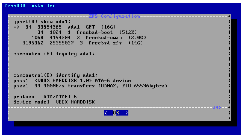
図2.22 ディスクの解析
