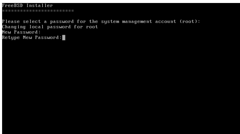
図2.29 root パスワードの設定
