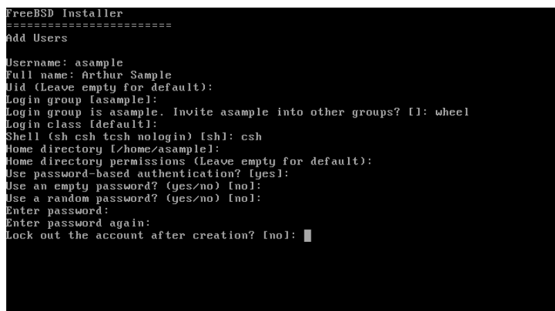
図2.49 ユーザ情報の入力
