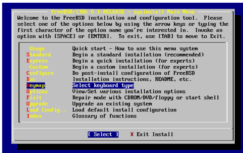
Afbeelding 2.8. Sysinstall hoofdmenu
