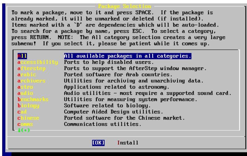
Afbeelding 2.47. Pakketcategorie kiezen
