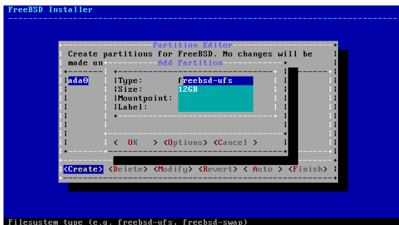
圖形 2.17. 手動建立分割區
