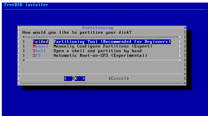
圖形 2.11. FreeBSD 10.x 或更新版本的磁碟分割選項
