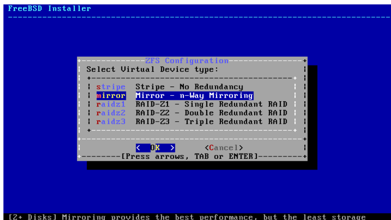
圖形 2.19. ZFS 儲存池類型
