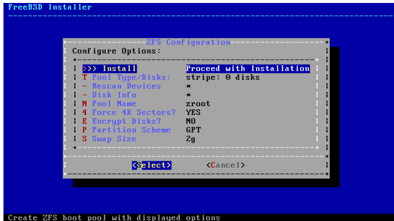
圖形 2.18. ZFS 磁碟分割選單
