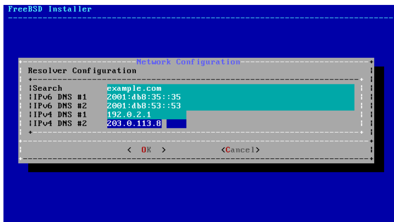
圖形 2.40. DNS 設定
