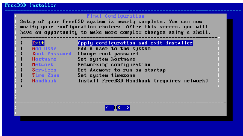
圖形 2.51. 最後設定
