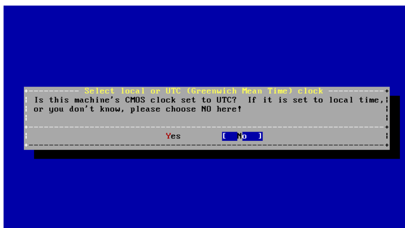
圖形 2.41. 選擇本地或 UTC 時鐘
