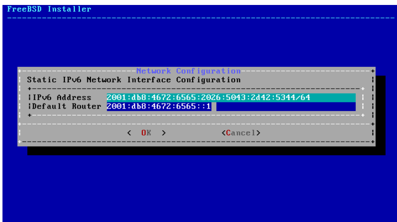
圖形 2.39. IPv6 靜態位置設定
